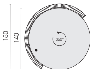
Element rund 360°-Drehfunktion Sonnenschirmaufnahme links 762DF*
