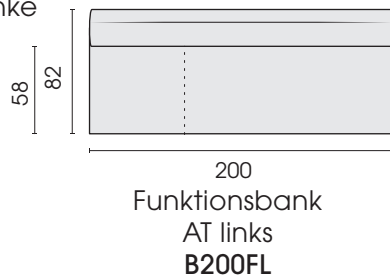
Frontansicht Typ B200FL
